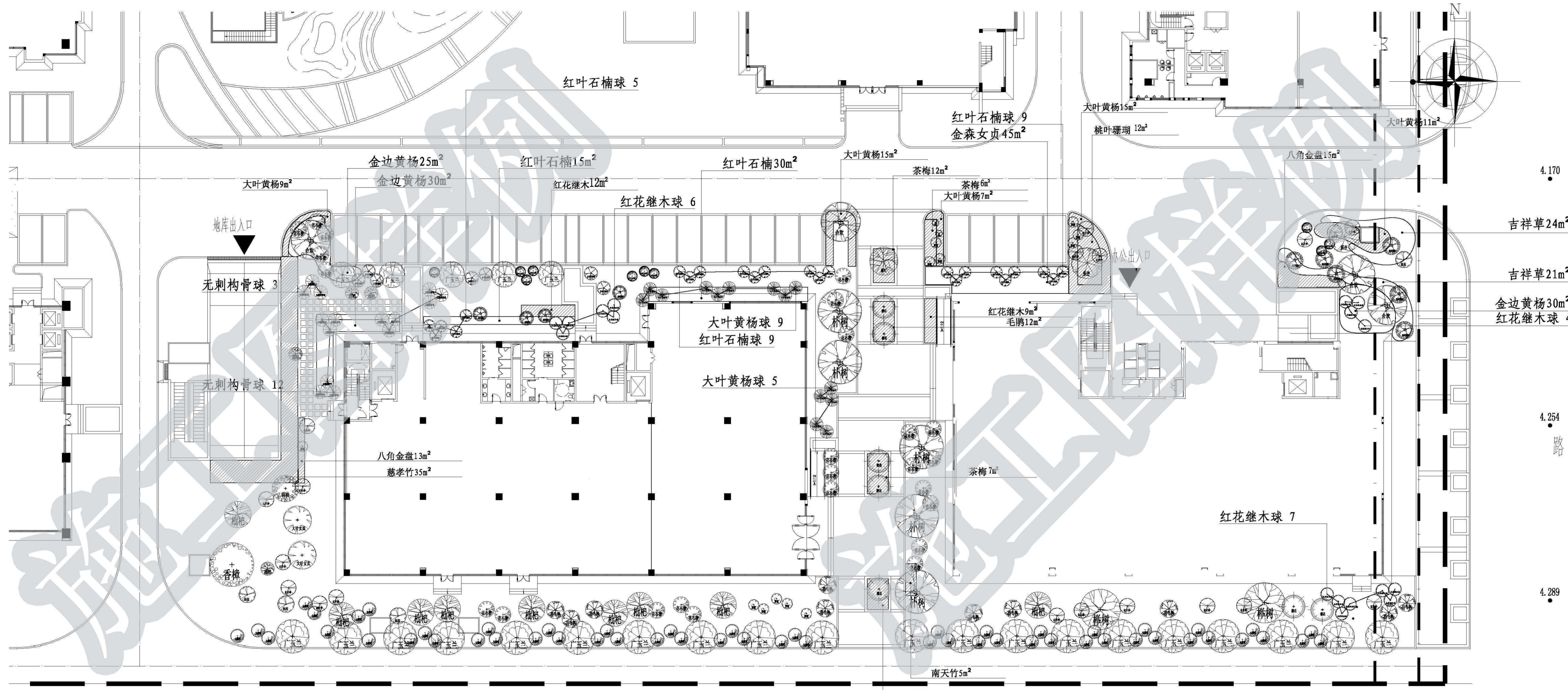
01 绿化平面图 SCALE 1:250
